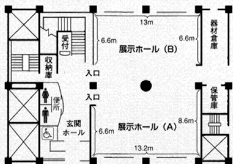
区民ギャラリー平面図（1階）
